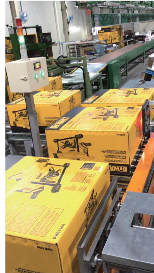
紙箱序號 OCR 辨識 OCR identification of carton serial numbers
